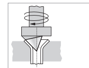
E-kontura konusa
